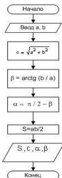
Рисунок 4 - Алгоритм примера 3
